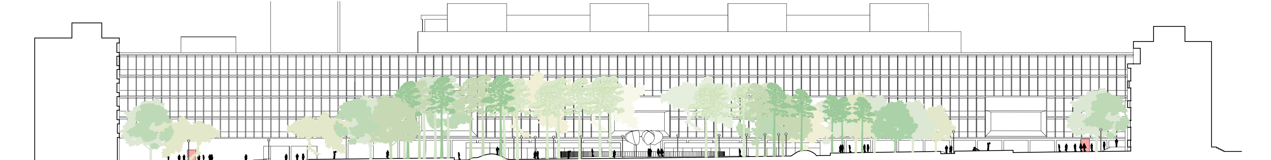
Rezopohľad námestím v mierke 1:500
